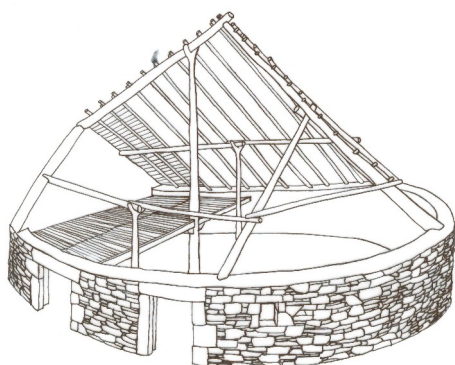
Sección constructiva.
